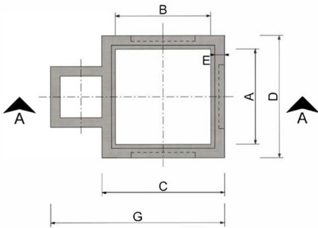
Pianta cod.00661
