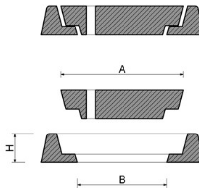
Sezioni A-A cod. 710-711-712
