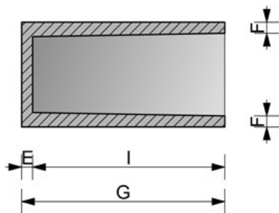
Sezione laterale cinerario
