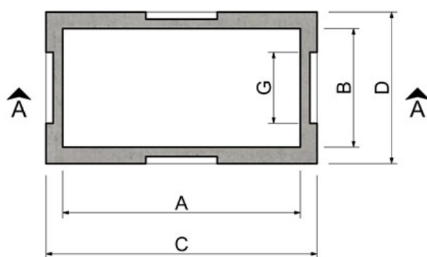
Pianta anello
